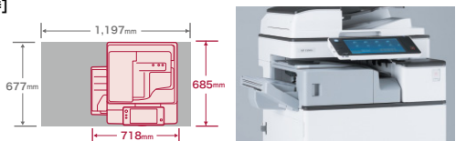
※写真はRICOH MP C5503Z SPFにオプションのインナーフィニッシャー SR3130を装着したものです。 ※転倒防止部材を含めない数値です。
