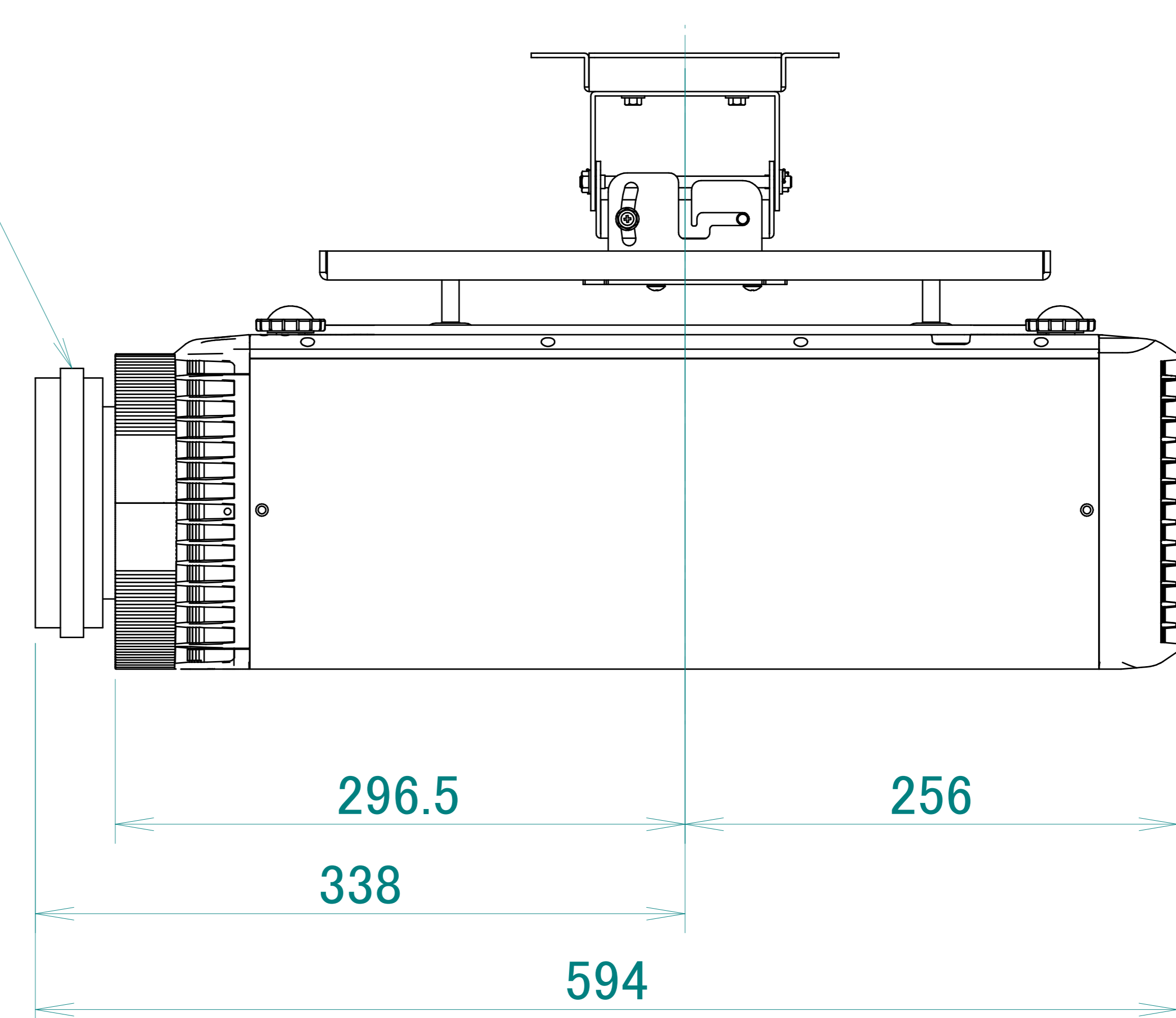
標準レンズ(タイプC3) Standard Lens(Type-C3)
